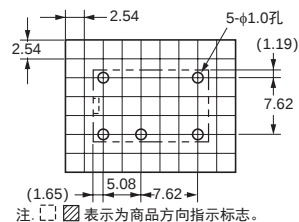
印刷基板加工尺寸 (BOTTOM VIEW) 尺寸公差为 \pm 0.1\text{mm}
