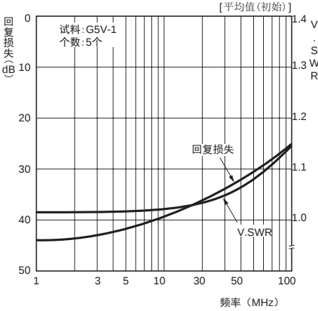
高频特性（回复损失、V.SWR） *1、*2
