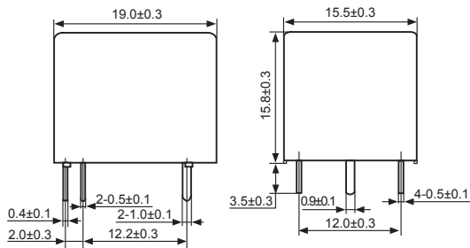
外形图
