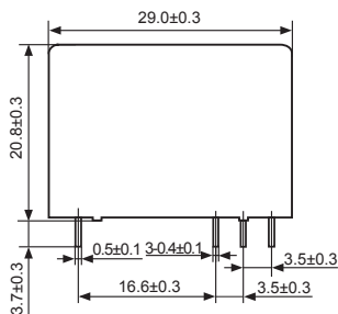
外形图
