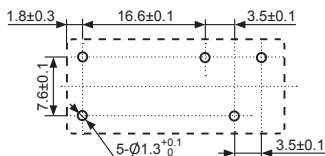
接线图 (底视图)
