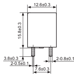
外形图
