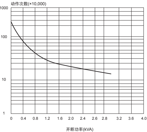
寿命曲线
