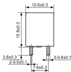
外形图
