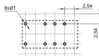
安装孔尺寸 (底视图)
