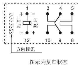
单线圈磁保持
