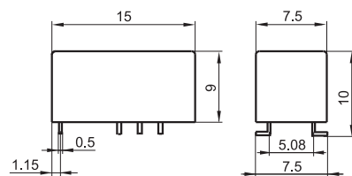
S1型: 短脚表面贴装型
