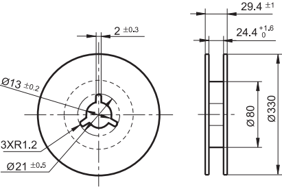
料盘外形图
