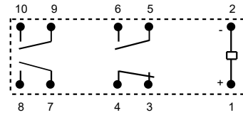
接线图
