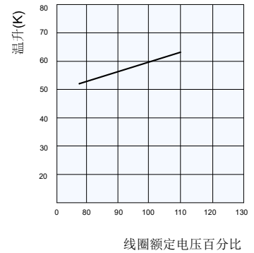
线圈温升
