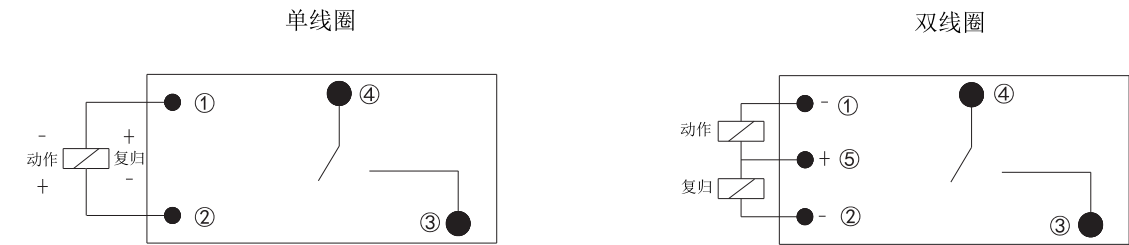
接线图 (底视图)
