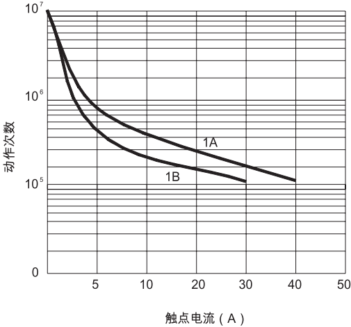
寿命曲线
