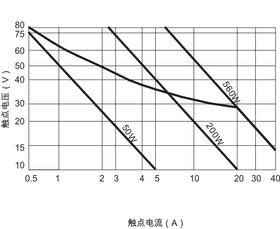
阻性负载下常开触点的灭弧能力
