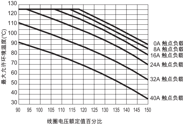
环境温度与线圈电压关系图
