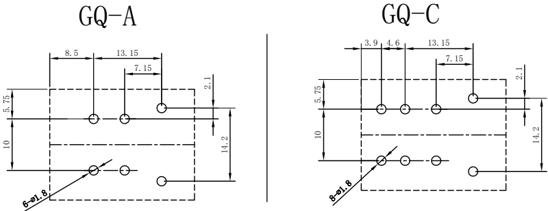
安装孔尺寸图（底视图）
