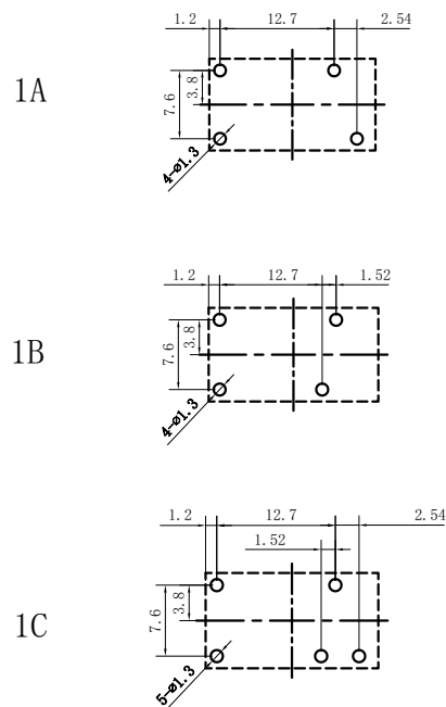
安装孔尺寸图 (底视图)
