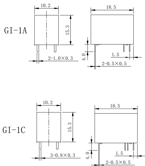
外形图
