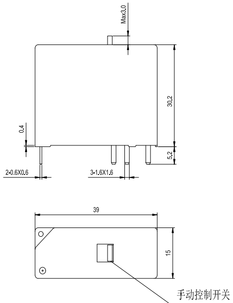
外形尺寸图
