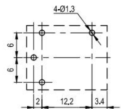
安装尺寸图
