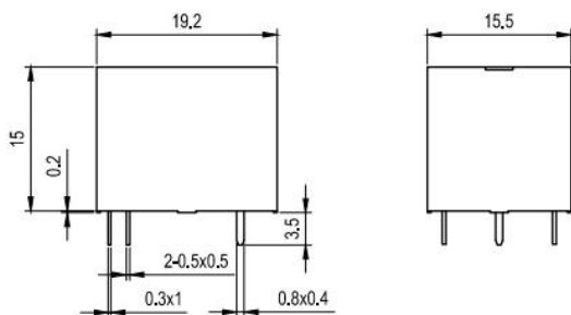
外形尺寸图
