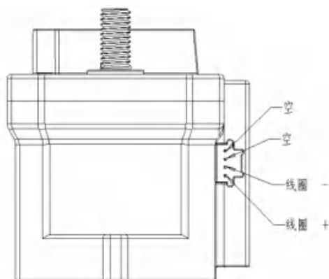
JCE-250P36BD, 不带辅助触头
