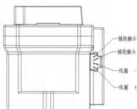
例: JCE-150P36AD5, 带辅助触头
