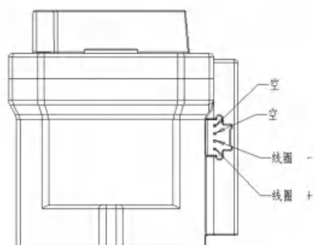
JCE-150P36BD5, 不带辅助触头
