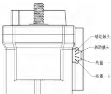
例: JCE-250P36AD, 带辅助触头
