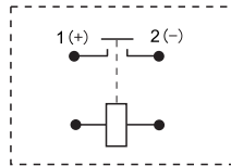
接线图
