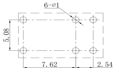
安装孔尺寸图 (底视图) P. C. B. Layout (bottom view)
