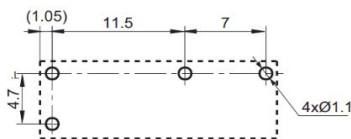
安装孔尺寸
