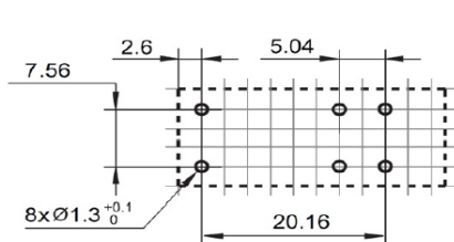
安装孔位图 (底视图)
