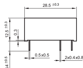
5mm引出脚间距
