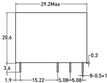
一组转换 1C
