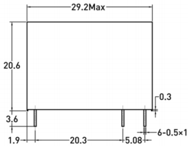
一组常开 1A
