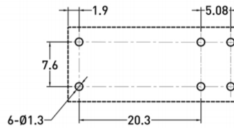
安装孔尺寸
