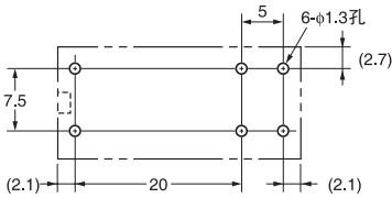
印刷基板加工尺寸 (BOTTOM VIEW)
