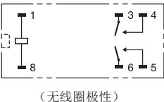
端子配置/内部接线图 (BOTTOM VIEW)
