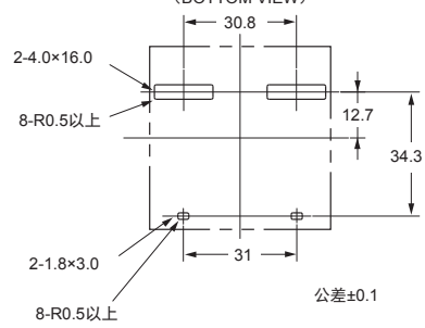
印刷电路板加工尺寸 (BOTTOM VIEW)
