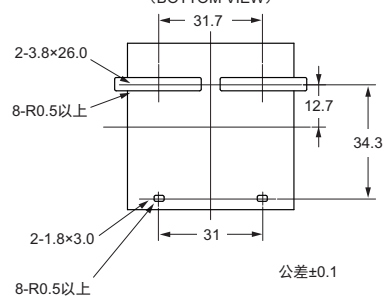
印刷电路板加工尺寸 (BOTTOM VIEW)
