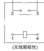
端子配置/内部接线图 (BOTTOM VIEW)
