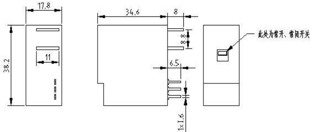
外形尺寸图： (双线圈)
