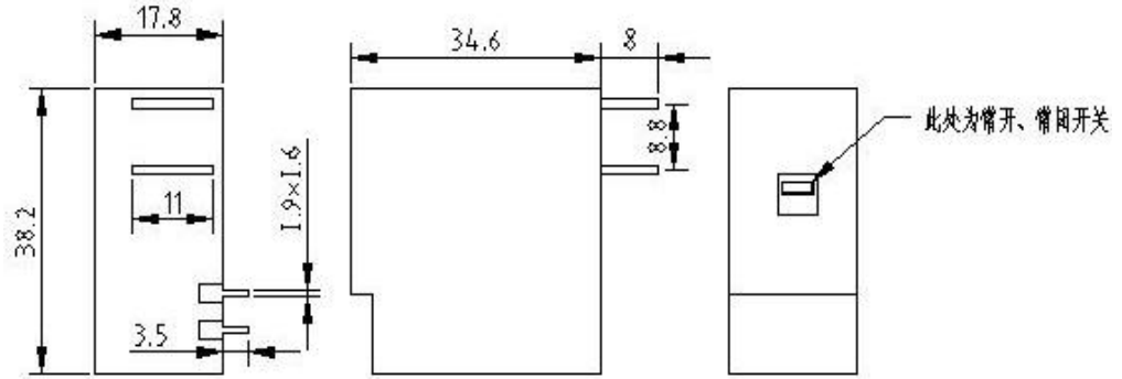
外形尺寸图： (单线圈)
