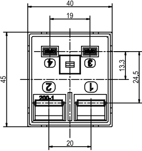
外形接线图
