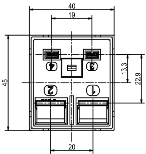
外形接线图
