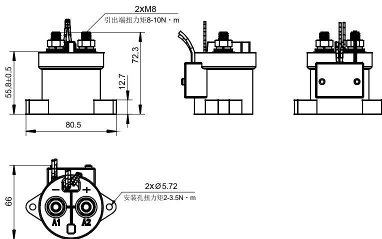
外形图
