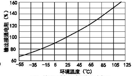
图3 输出压降与环境温度关系曲线
