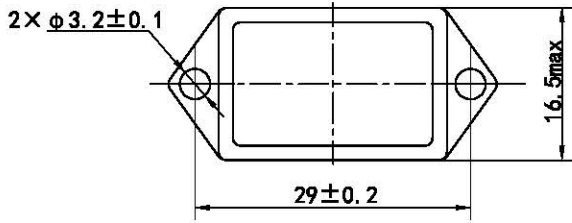
a) 外形、安装尺寸与引出端型式1
