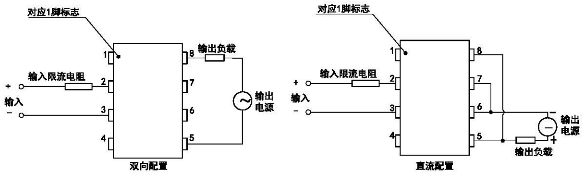
d) 俯视接线图
