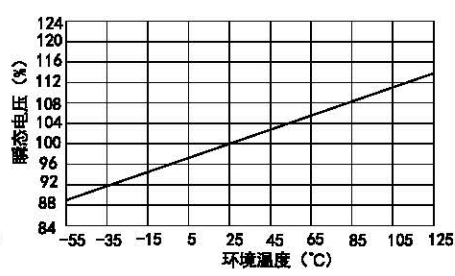
图6 归一化瞬态电压与环境温度关系曲线
