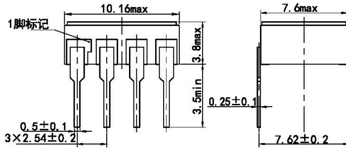
a) 外形、安装尺寸与引出端型式 1 (DIP8 型)
