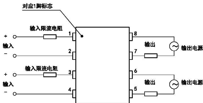
d) 俯视接线图
