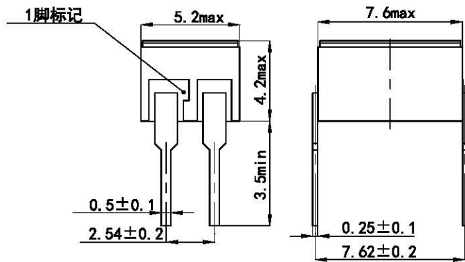
a) 外形、安装尺寸与引出端型式 1 (DIP4 型)
