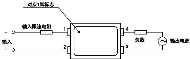
d) 俯视接线图
