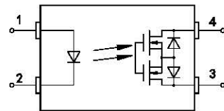
e) 内部电路图
