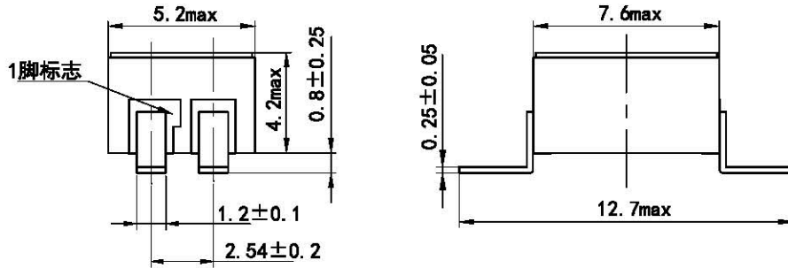
b) 外形、安装尺寸与引出端型式 2 (SMD4 型)
