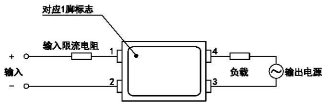
d) 俯视接线图
