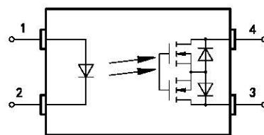
e) 内部电路图
