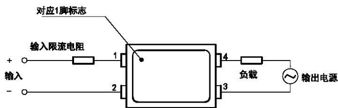
d) 俯视接线图
