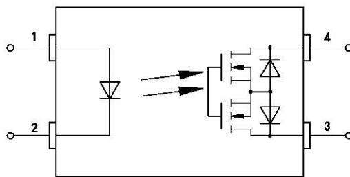
e) 内部电路图
