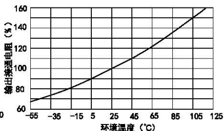
图3 归一化输出接通过阻与环境温度关系曲线
