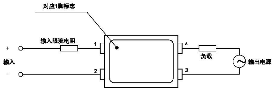
b) 俯视接线图
