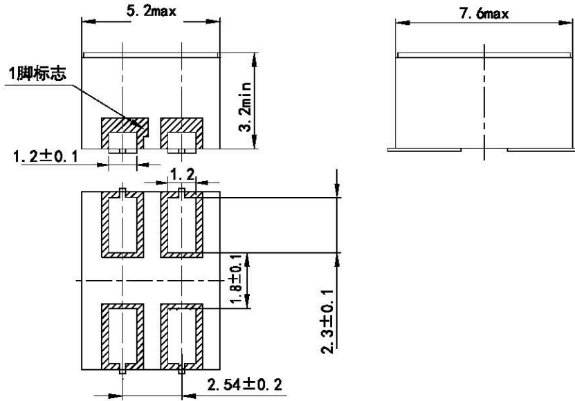
a) 外形、安装尺寸与引出端型式 (LCC4 型)
