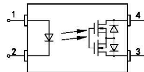
e) 内部电路图
