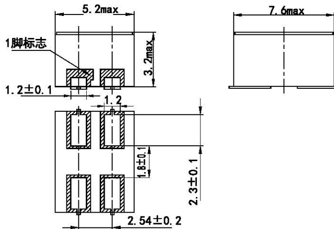
b) 外形、安装尺寸与引出端型式 2 (SMD4 型)
