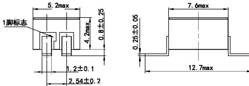
a) 外形、安装尺寸与引出端型式 1 (DIP4 型)
