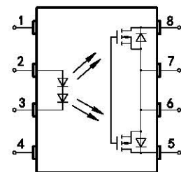
e) 内部电路图
