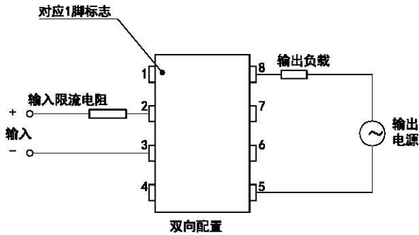
d) 俯视接线图
