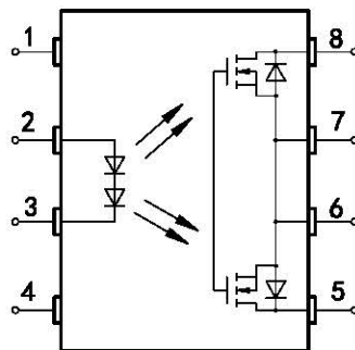
e) 内部电路图
