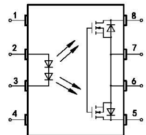
e) 内部电路图
