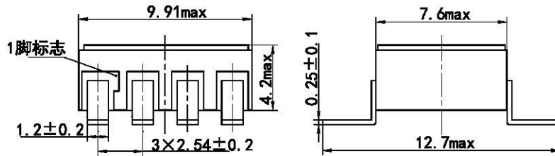
a) 外形、安装尺寸与引出端型式 1 (DIP8 型)
