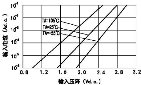
图4 输入电流与输入电压关系曲线
