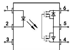
e) 内部电路图
