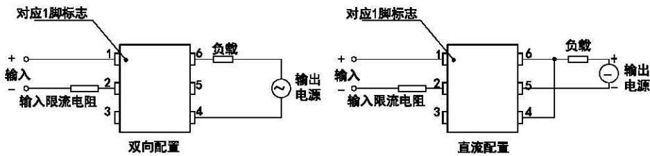
d) 俯视接线图
