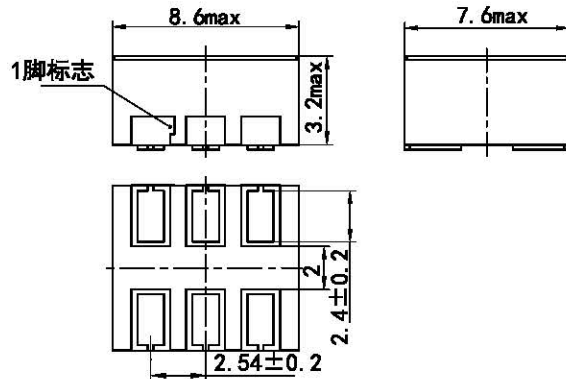
c) 外形、安装尺寸与引出端型式 3 (LCC6 型)
