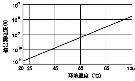
图5 输出漏电流与环境温度关系曲线
