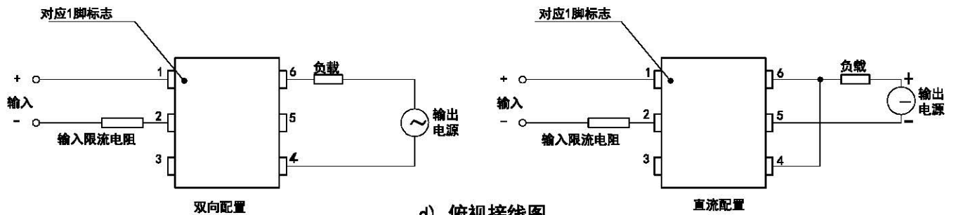
d) 俯视接线图
