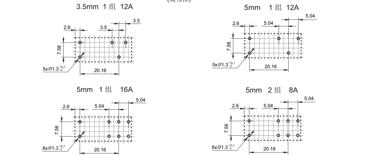
安装孔尺寸 (底视图)
