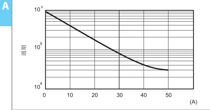
F 67 - 電氣壽命與觸點電流 (AC1/AC7a 負載)
