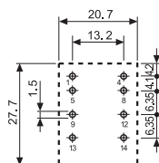
PCB銅箔側視圖
