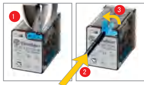
可鎖定測試按鈕和機械式指示器 (0010、0040、0050、0054、0070、0074、0090、0094)
