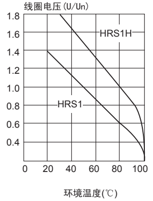
线圈工作范围曲线
